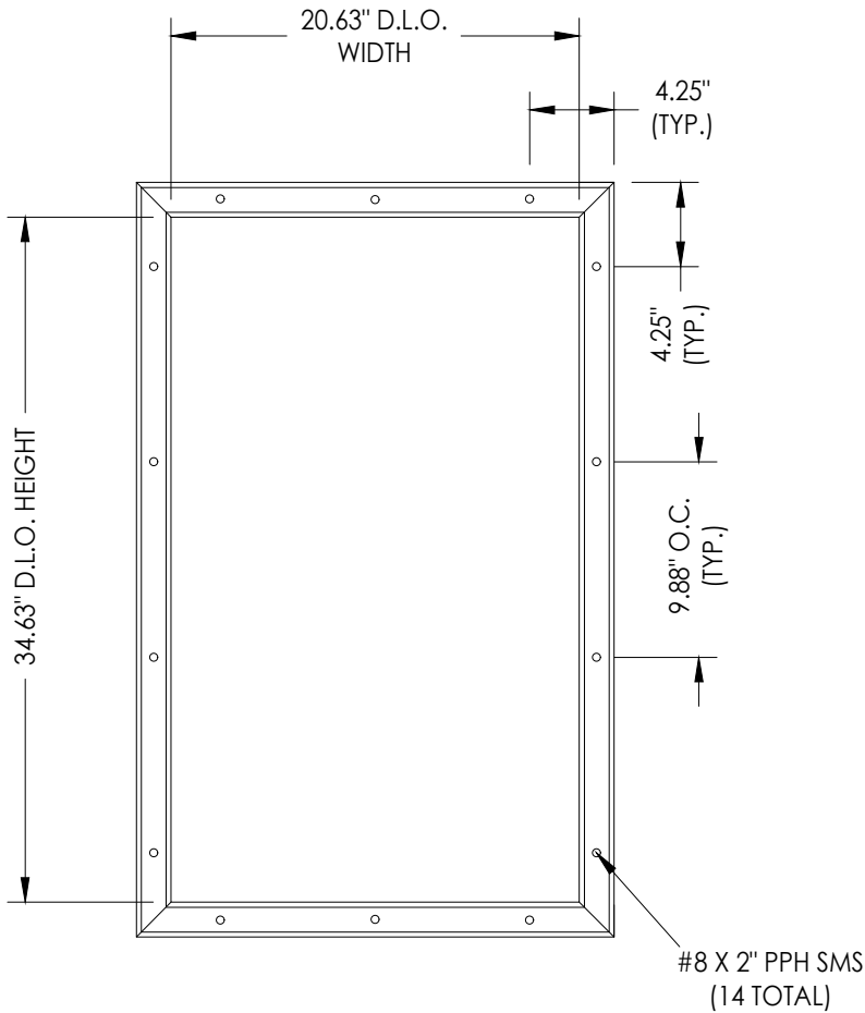
ODL LITE FRAME
